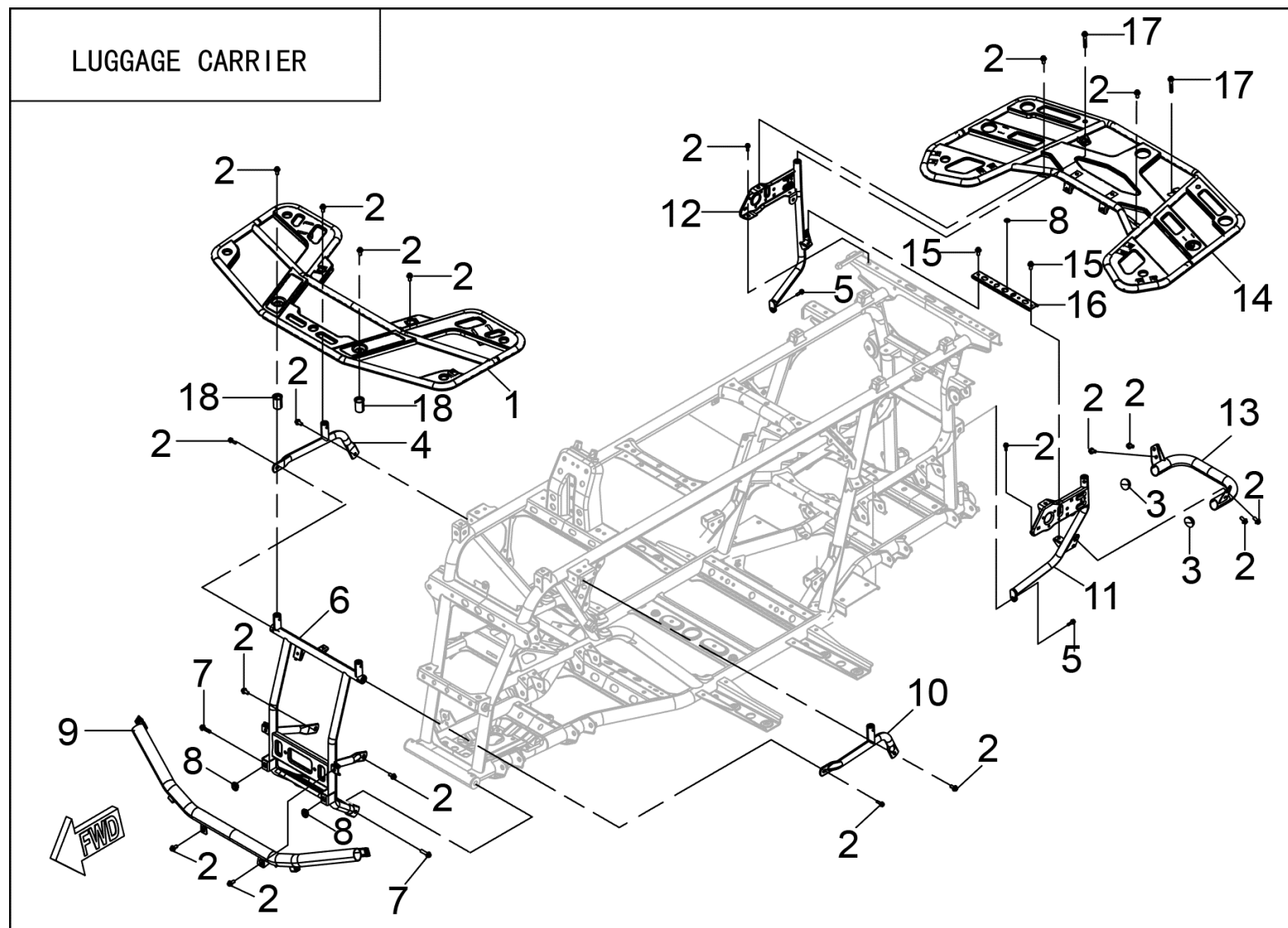
FIGUR 23 - BAGAGEBÆRER
