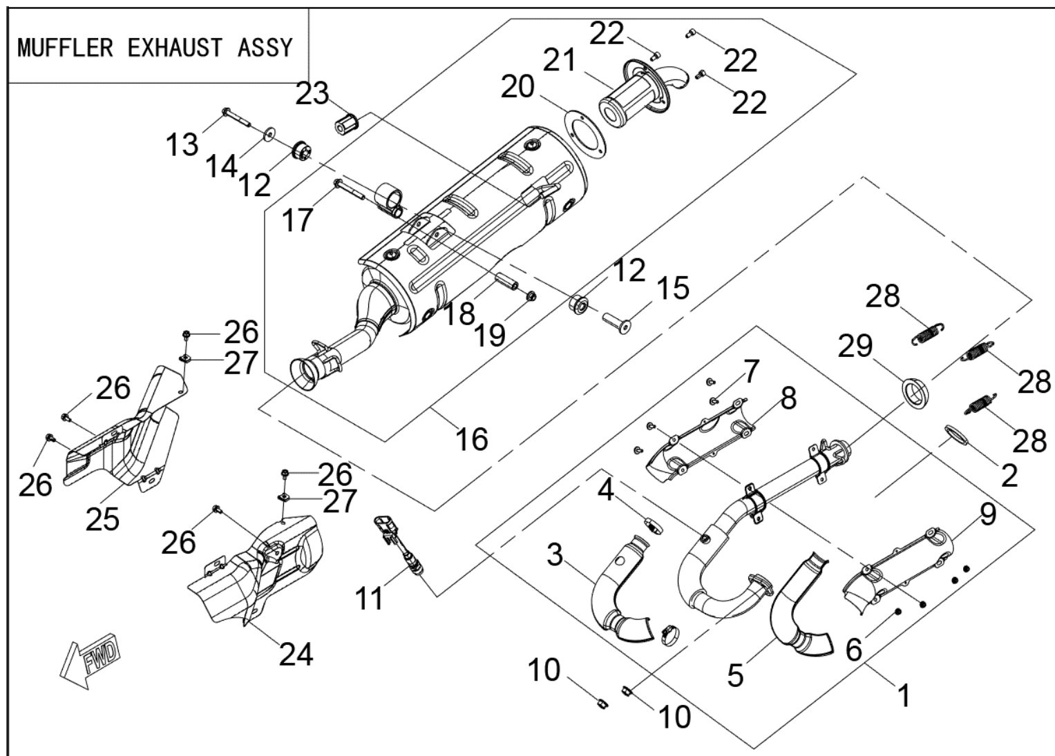
FIGUR 4 – UDSTØDNING / LYDDÆMPER
