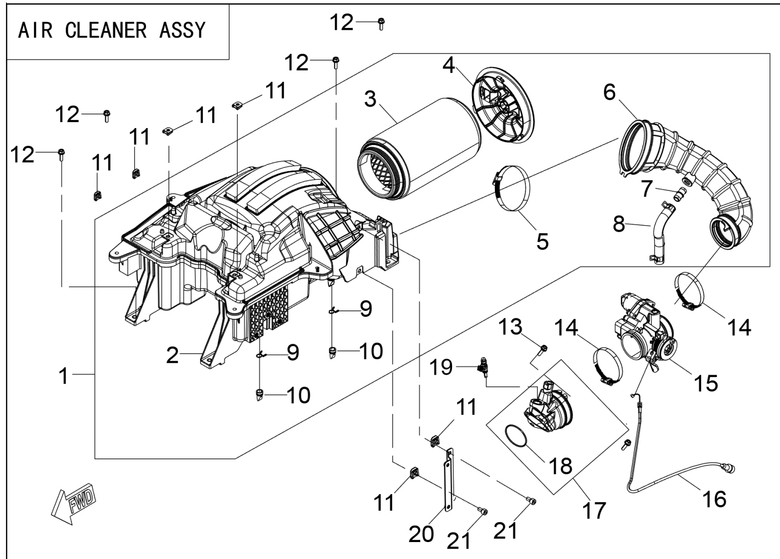
FIGUR 3 – LUFTFILTER
