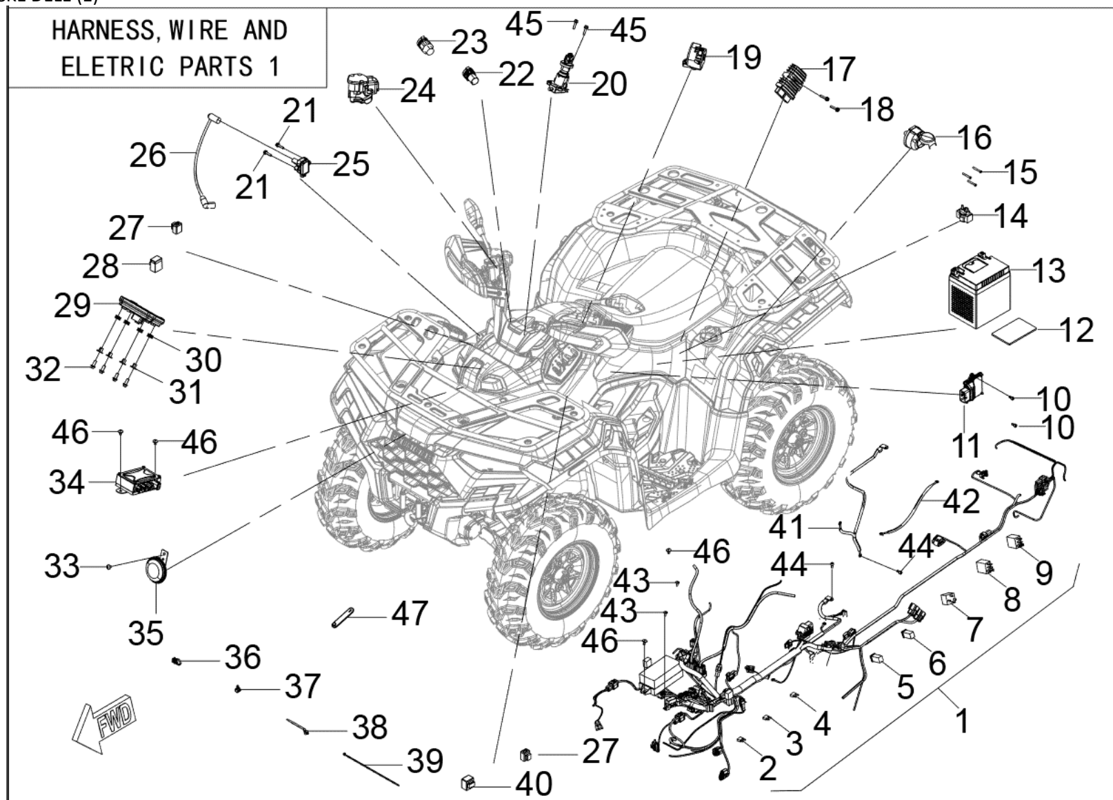
FIGUR 9 – ELEKTRISKE DELE (1)
