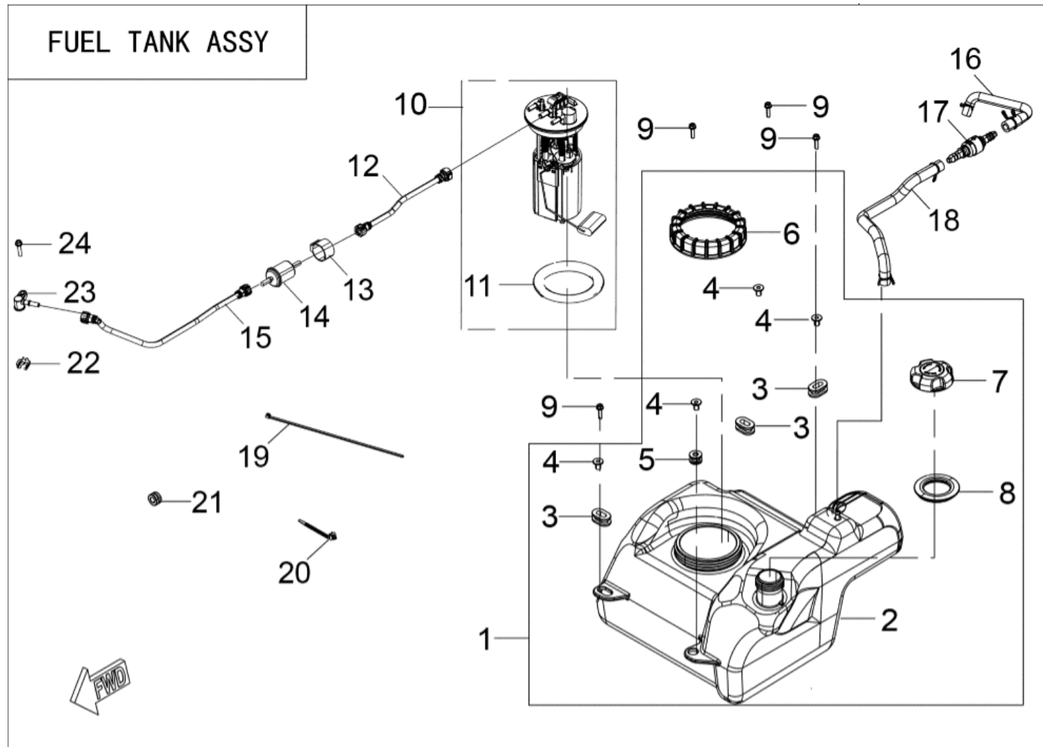
FIGUR 2 – BRÆNDSTOFTANK
