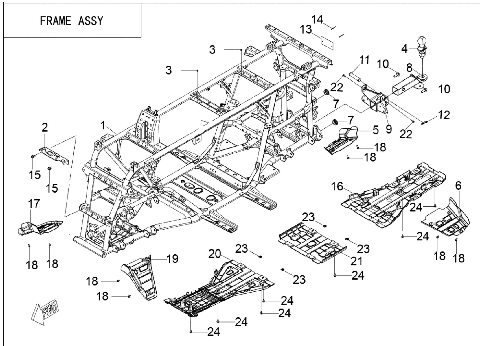
FIGUR 18 - STEL
