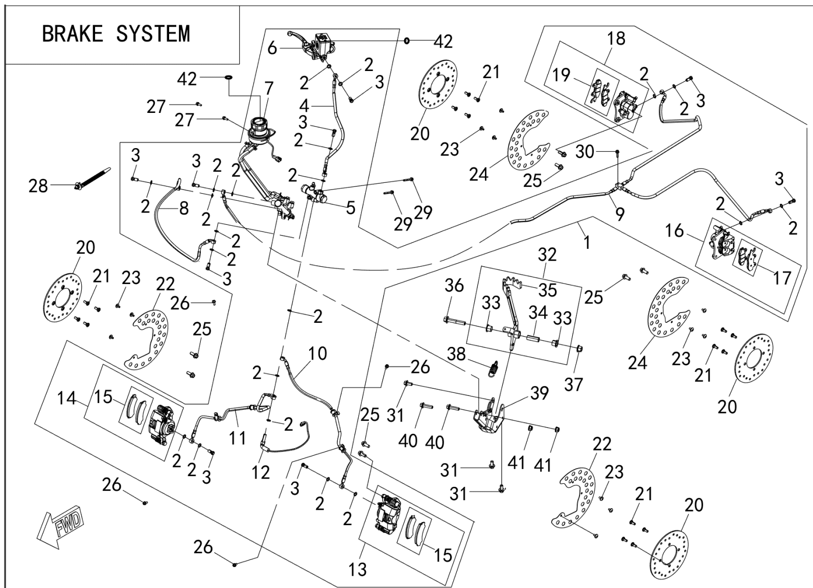
FIGUR 13 – BREMSESYSTEM
