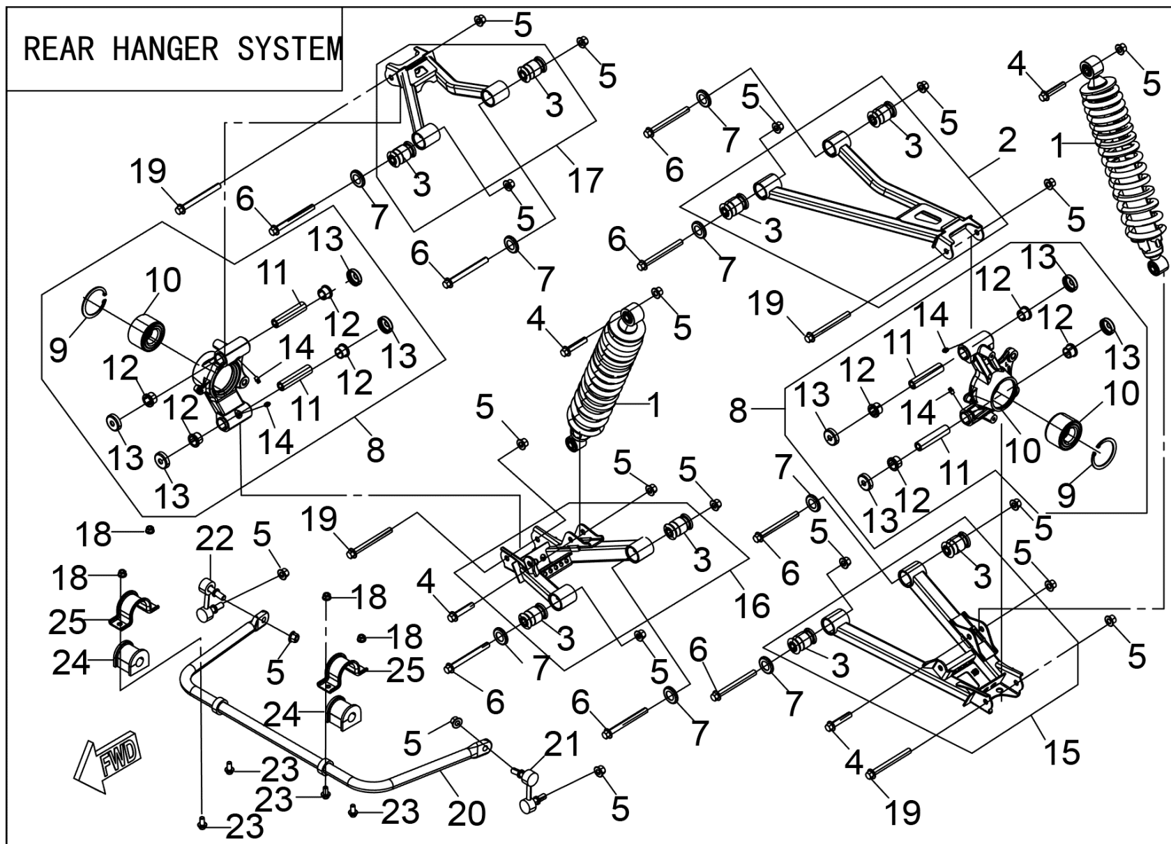
FIGUR 20 – BAGTØJ
