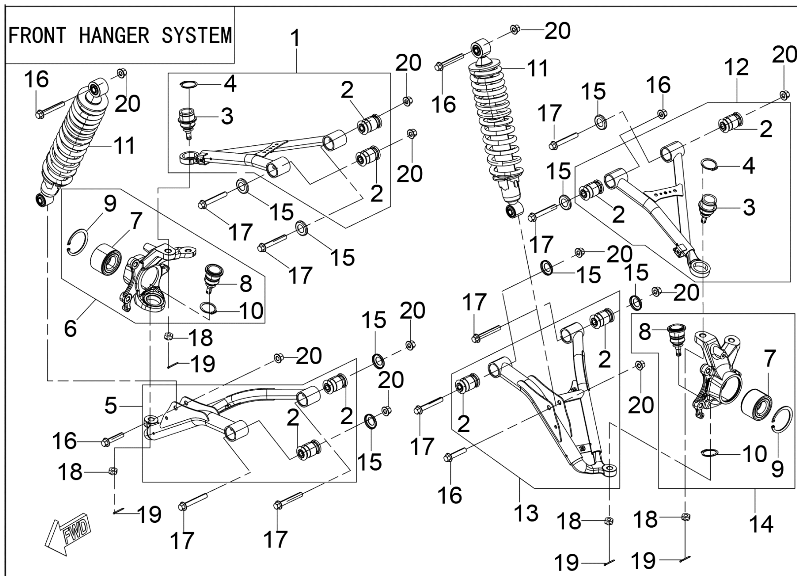
FIGUR 19 – FORHJULSOPHÆNG
