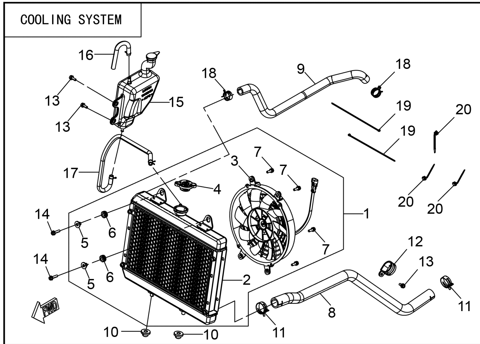
FIGUR 1 – KØLESYSTEM
