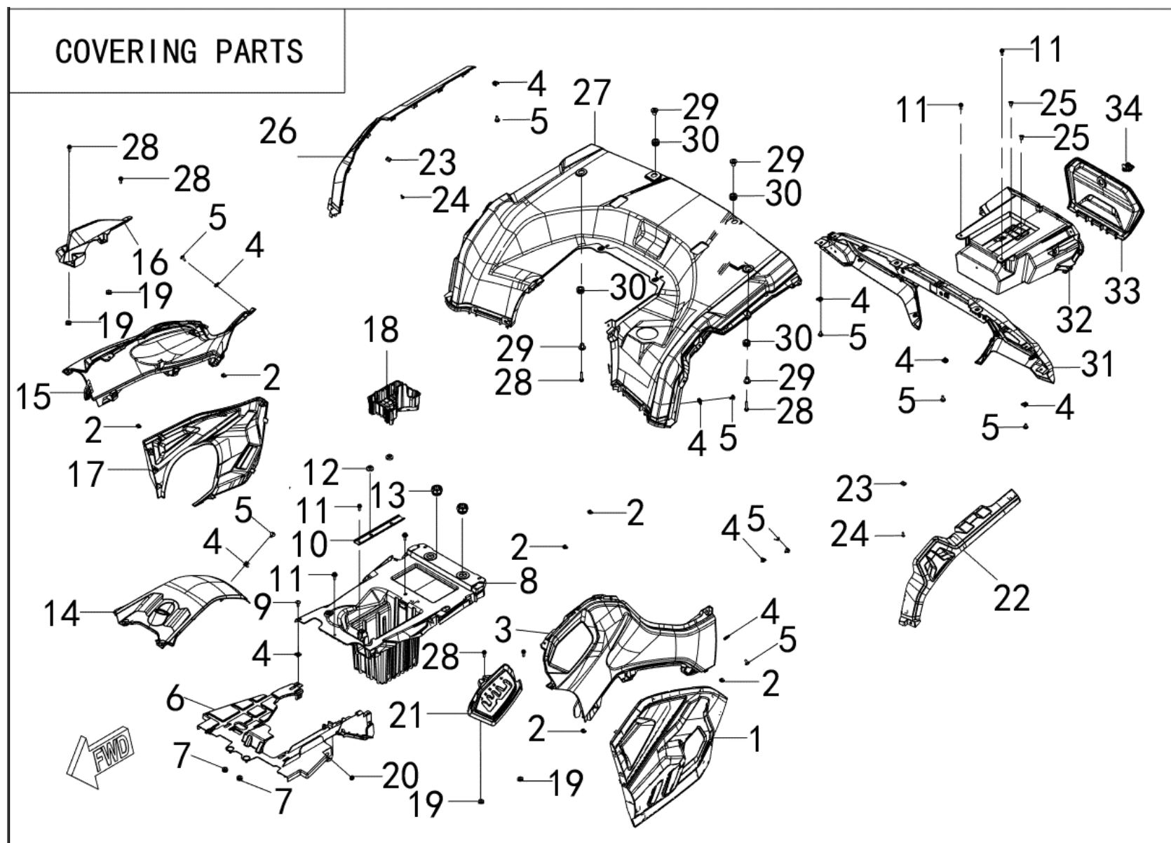
FIGUR 26 - SKÆRMDELE
