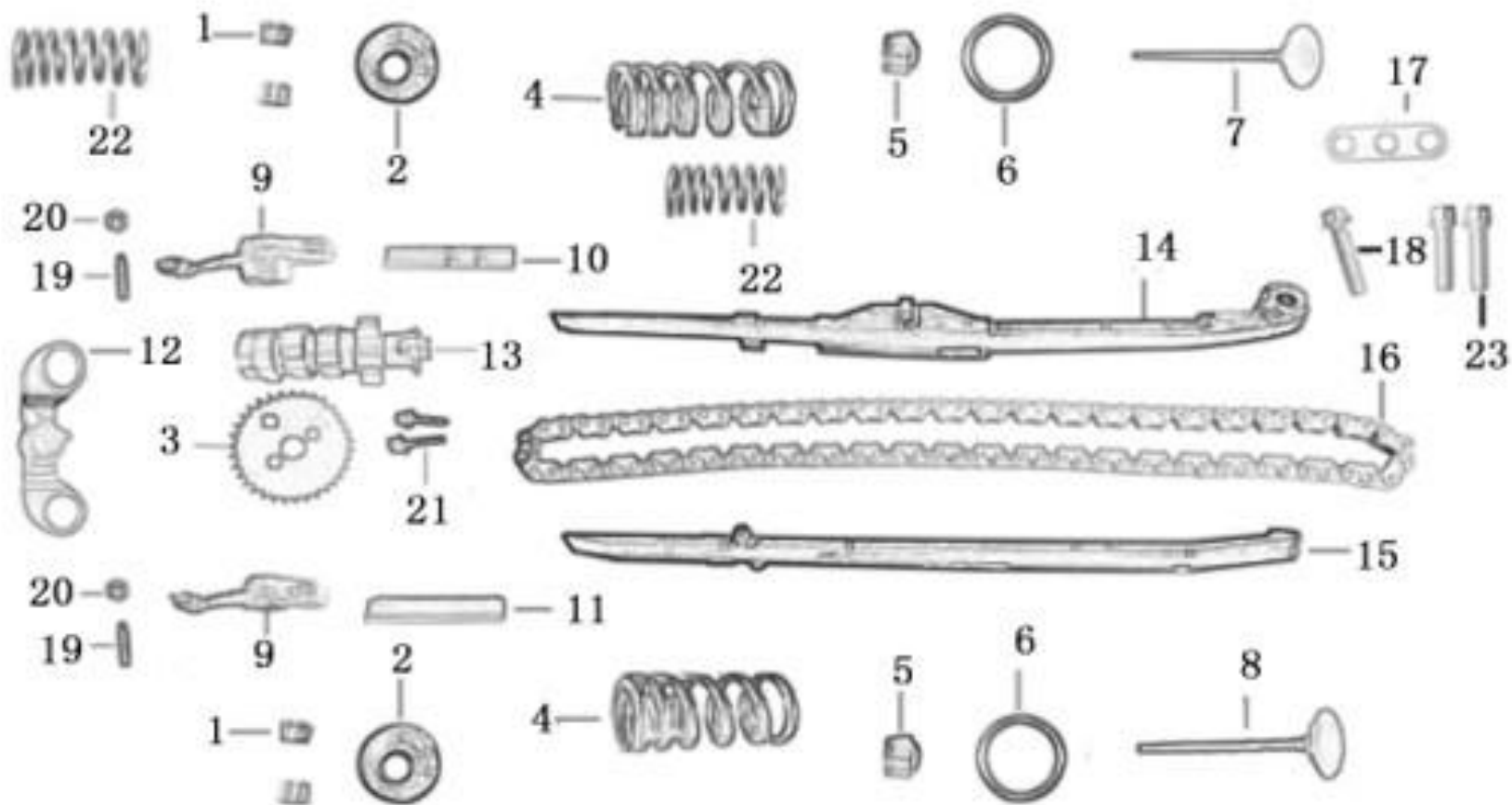
FIGUR E3 – VENTIL / VALVE
